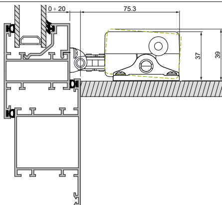
Apertura a sporgere con staffe abbaino
